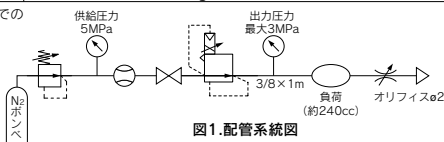
図1. 配管システム図
