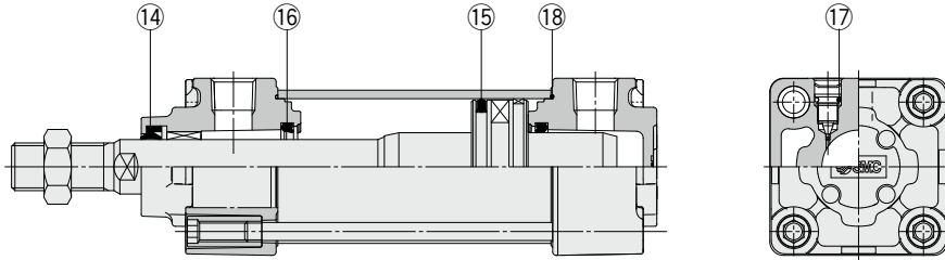
※上図はMB-Zシリーズの構造図です。 番号はホームページWEBカタログ MB-Zシリーズの構造図と同じになっています。
